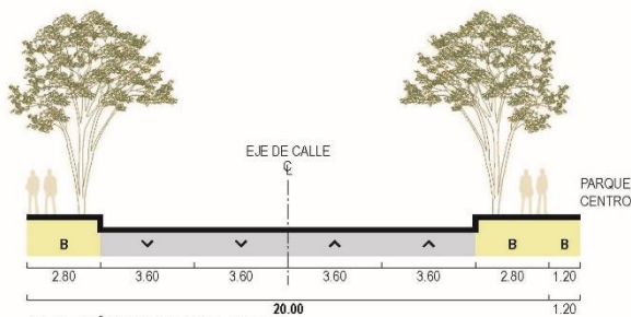
SECCIÓN TIPO VIII, SAUCE
