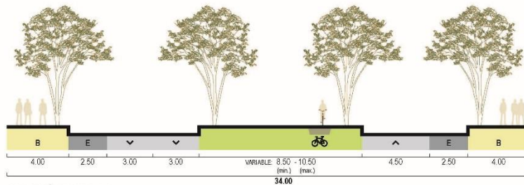
SECCIÓN TIPO III
