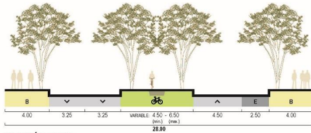
SECCIÓN TIPO I
