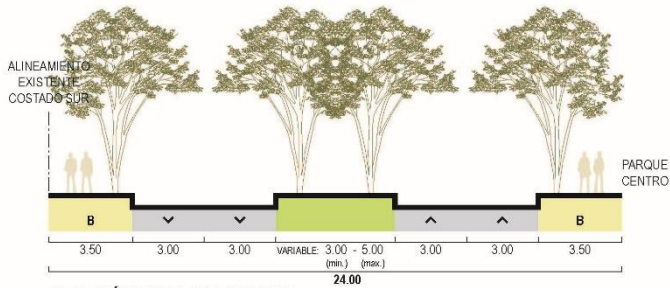
SECCIÓN TIPO V, LEONES
