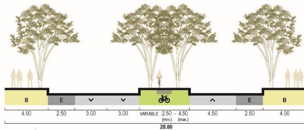
SECCIÓN TIPO II
