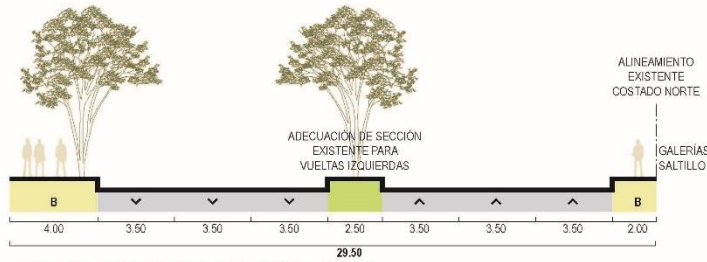
SECCIÓN BOULEVARD GALERÍAS, TIPO G
