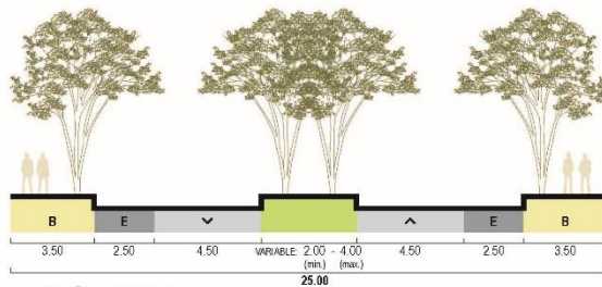
SECCIÓN TIPO IV
