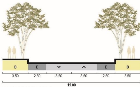
SECCIÓN TIPO VI
