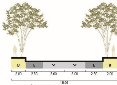
SECCIÓN TIPO VII
